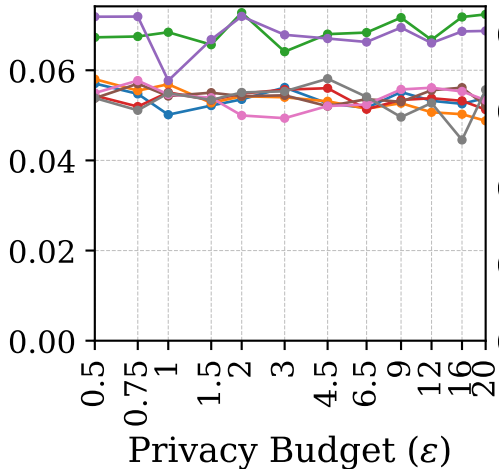
LastFM
