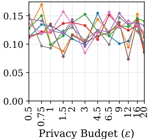
Facebook
