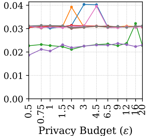
Brightkite
